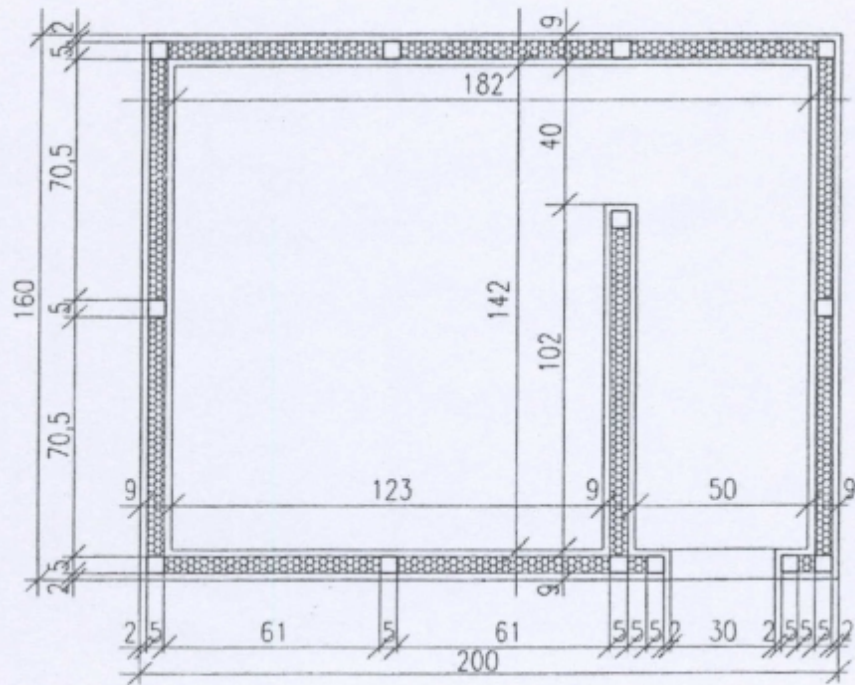
RZUT BUDY
