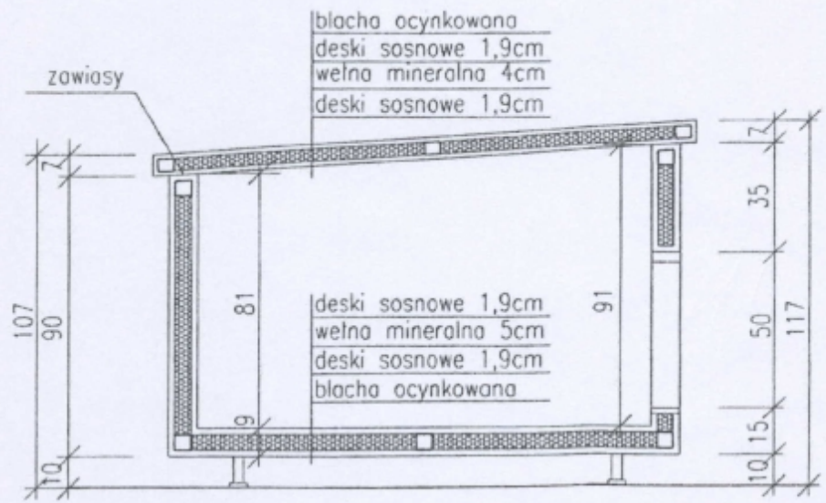
PRZEKRÓJ
