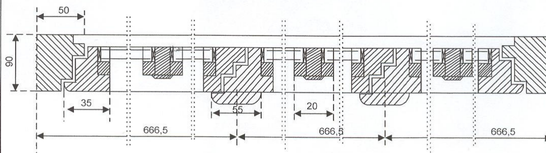
Przekrój A-A
