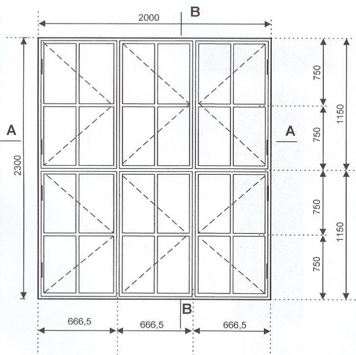
Okno zespolone dwuszybowe sztuk 6
