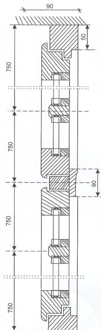
Przekrój B-B
