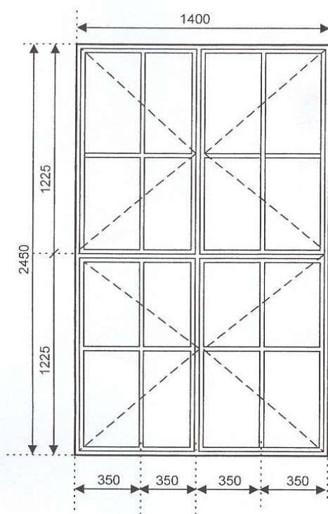
Okno skrzynkowe pojedyncze sztuk 9
